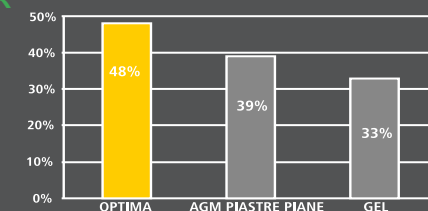
LIVSCYKEL VS URLADDNING FÖR OPTIMA BATTERIER
