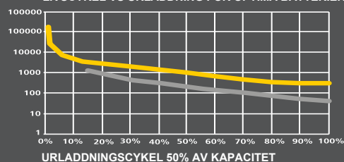
LIVSCYKEL VS URLADDNING FÖR OPTIMA BATTERIER
